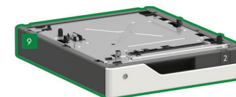
9 Bac verrouillable de 250 feuilles 80 x 428 x 510 mm
