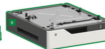
8 Bac verrouillable de 550 feuilles 110 x 428 x 510 mm
